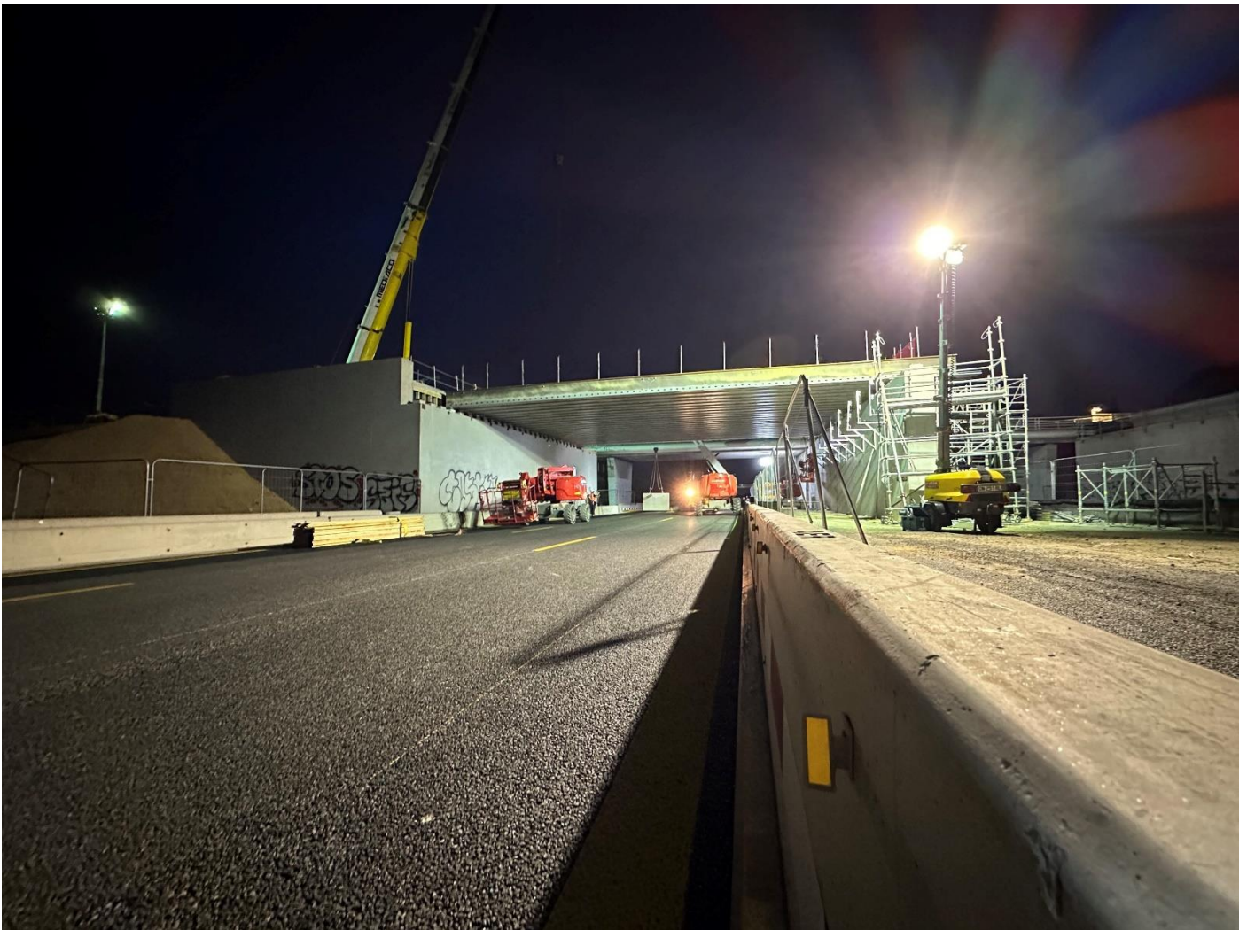
La pose des poutres métalliques qui constituent le partie plane du futur pont sont en cours. (photo : VINCI Autoroutes)
