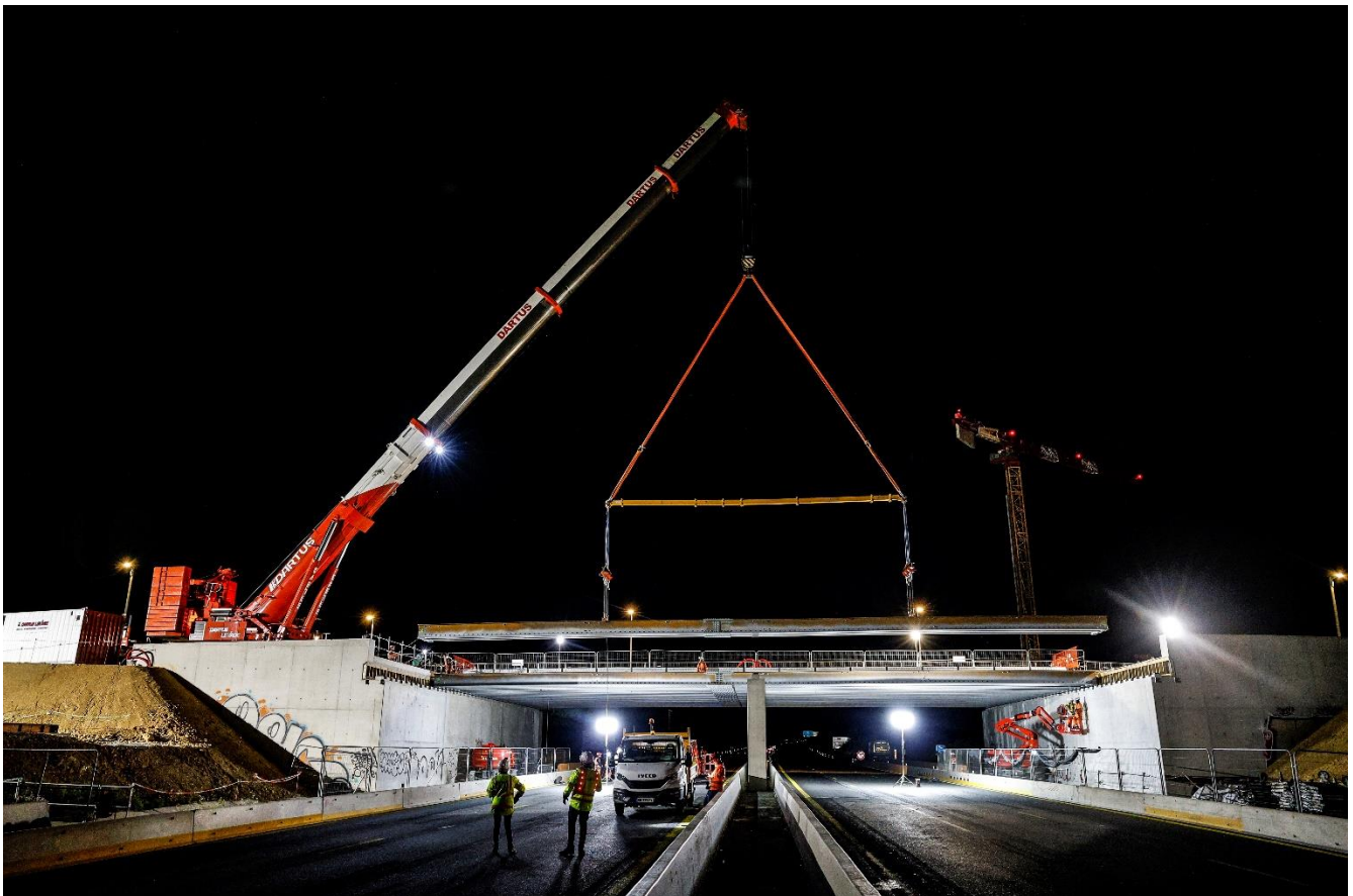
Pose des poutres métalliques qui constituent la partie plane du futur pont. (Photo : Alain TENDERO)
